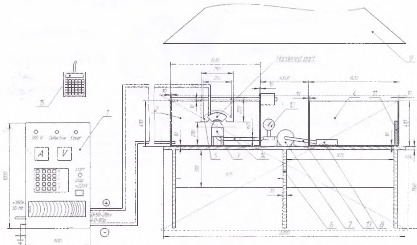
2 сурет – ЭПМ кондырғысын монтаждау және демонтаждау, үлгілерді/бөлшектерді реттеу.
