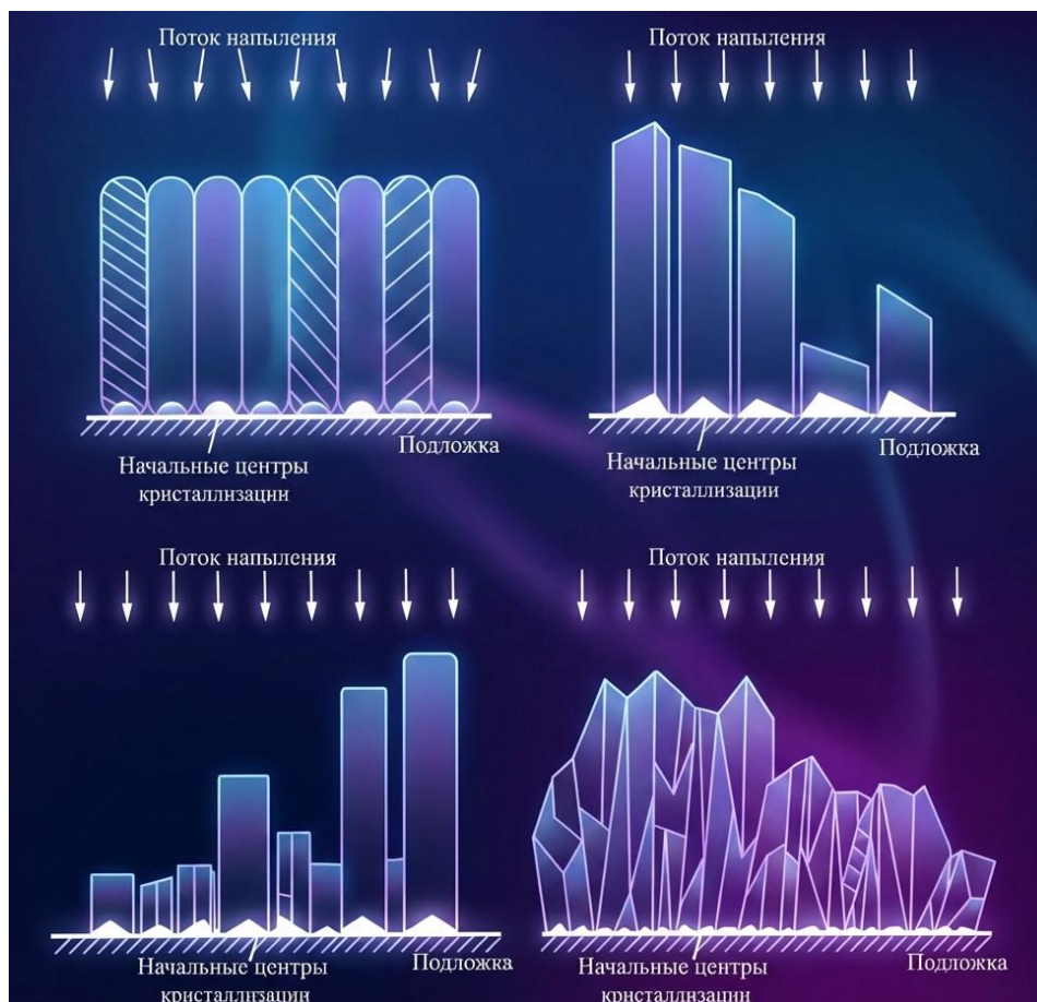
Рисунок 2.12 - Двумерные структуры роста, построенные для нескольких экстремальных случаев диффузии адатомов по поверхности. а) Исключена диффузия, все частицы конденсируются без потерь. б) Диффузия отсутствует, но эффективность осаждения определяется типом поверхности. в) Реализован режим бесконечной диффузии. г) Бесконечная диффузия в сочетании с регулярным повторным нуклеационным процессом
