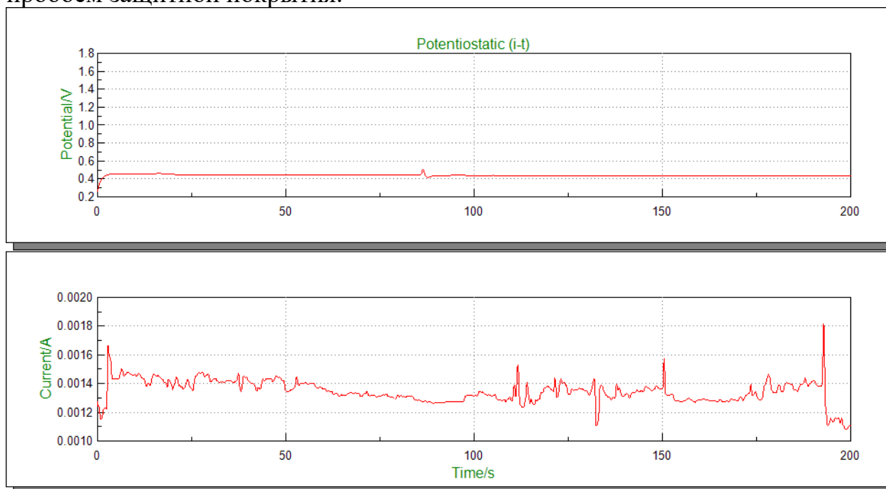
Рисунок 4.9 - Зависимость потенциала и тока от времени для покрытия TaCu
