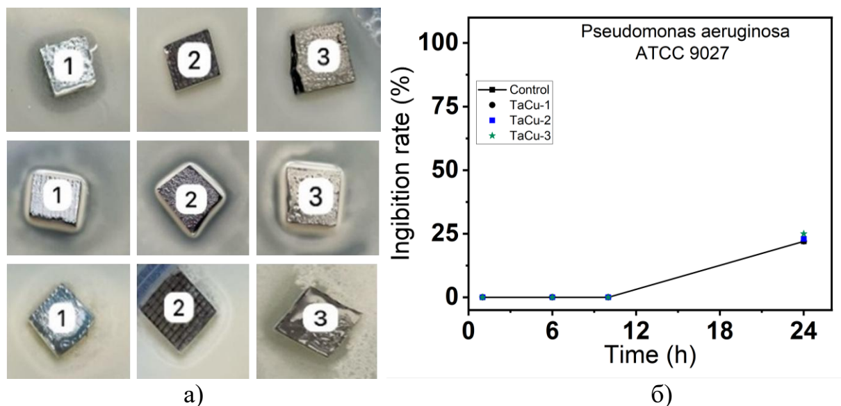
Рисунок 4.11 – а) фотографии опытных образцов б) зависимость антибактериальной активности покрытий TaCu от технологических режимов осаждения
