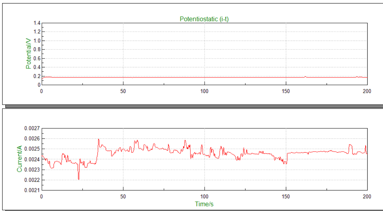
Рисунок 4.8 - Зависимость потенциала и тока от времени для покрытия NbCu
